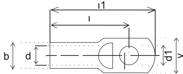
Bimetalik Kablo Pabucu Bimetallic Cable Lug
