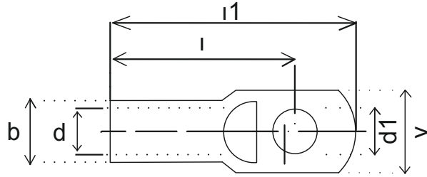
Alüminyum Kablo Pabucu Aluminium Kablo Pabucu
