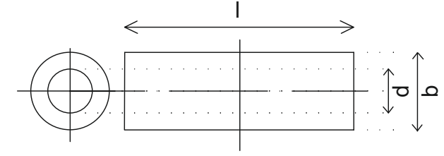
Bimetalik Konnektör Bimetallic Connector
